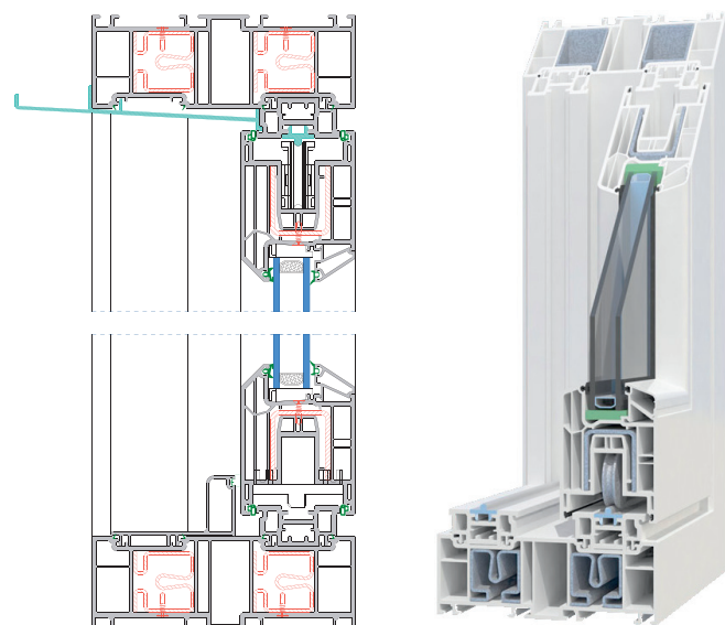
Sección vertical Elevadora
